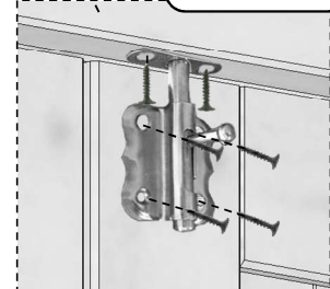
INSIDE 6x \varnothing 3,5 \times 35
